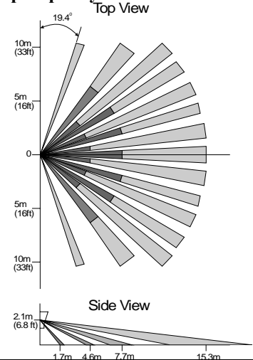
Рис. 2 - Диаграмма направленности суперширокоугольной линзы
