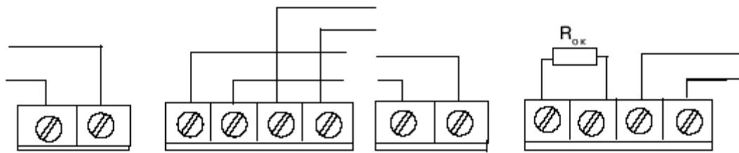
+ ШС - + ШС - Доступ + ШС - + ШС - Доступ а) при включении в разрыв ШС б) При включении на конце ШС
