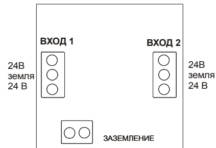
Рисунок 1б – АЛЬБАТРОС 24/70
