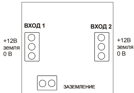
Рисунок 1а – АЛЬБАТРОС 12/70
