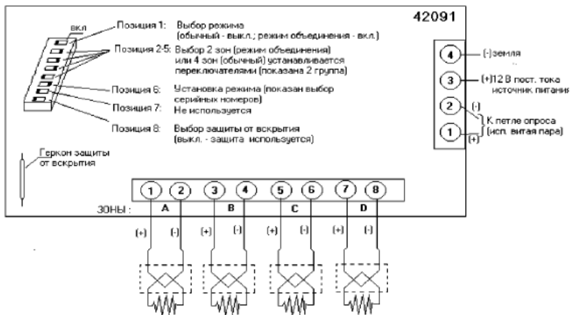
Рис. 1. Схема соединений
