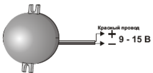
Рис.2 Схема подключения ПКИ - ОС1.
