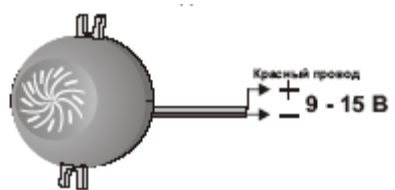
Рис.2 Схема подключения ПКИ-СП12.
