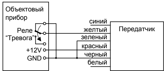
Рис. 3. Примеры монтажа передатчика
