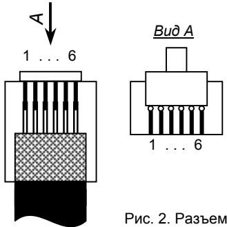
Рис. 2. Разъем
