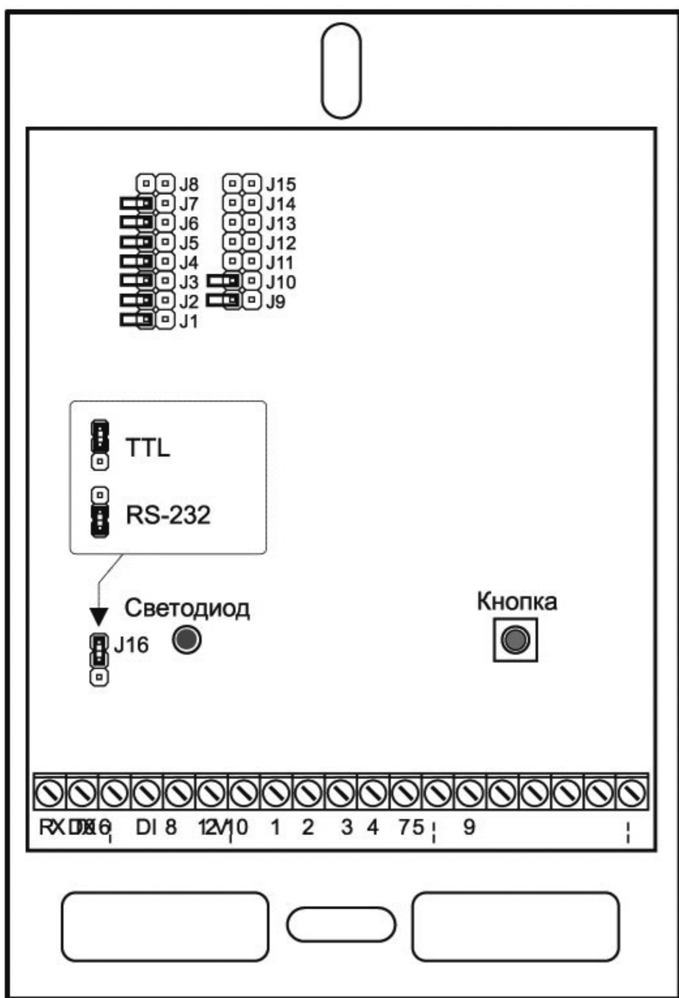
Монтажная схема расширителя
