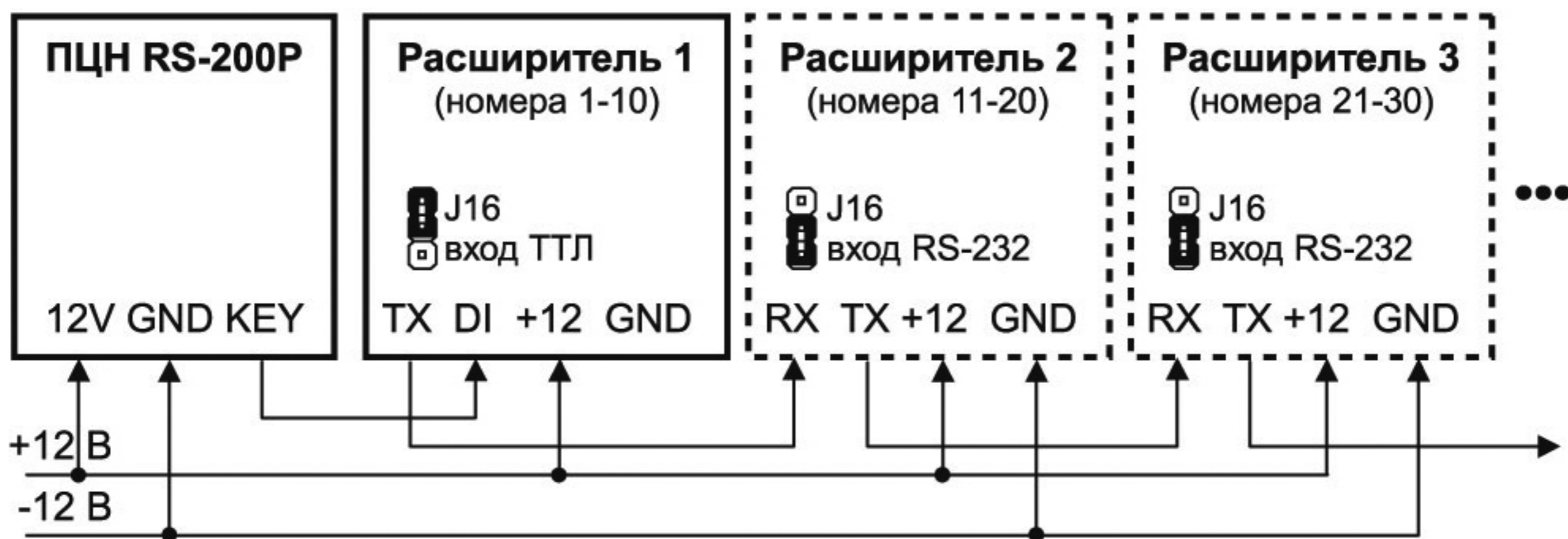
Подключение расширителя к ПЦН RS-200P (до 16 шт.)
