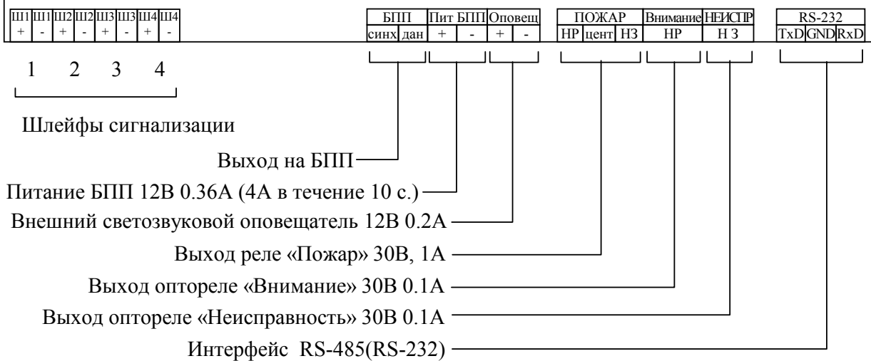
Назначение контактов отсека коммутации БПК
