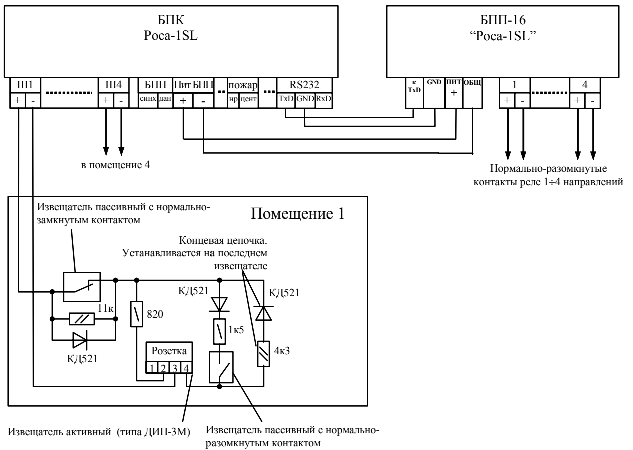
Типовая схема подключения БПП-16
