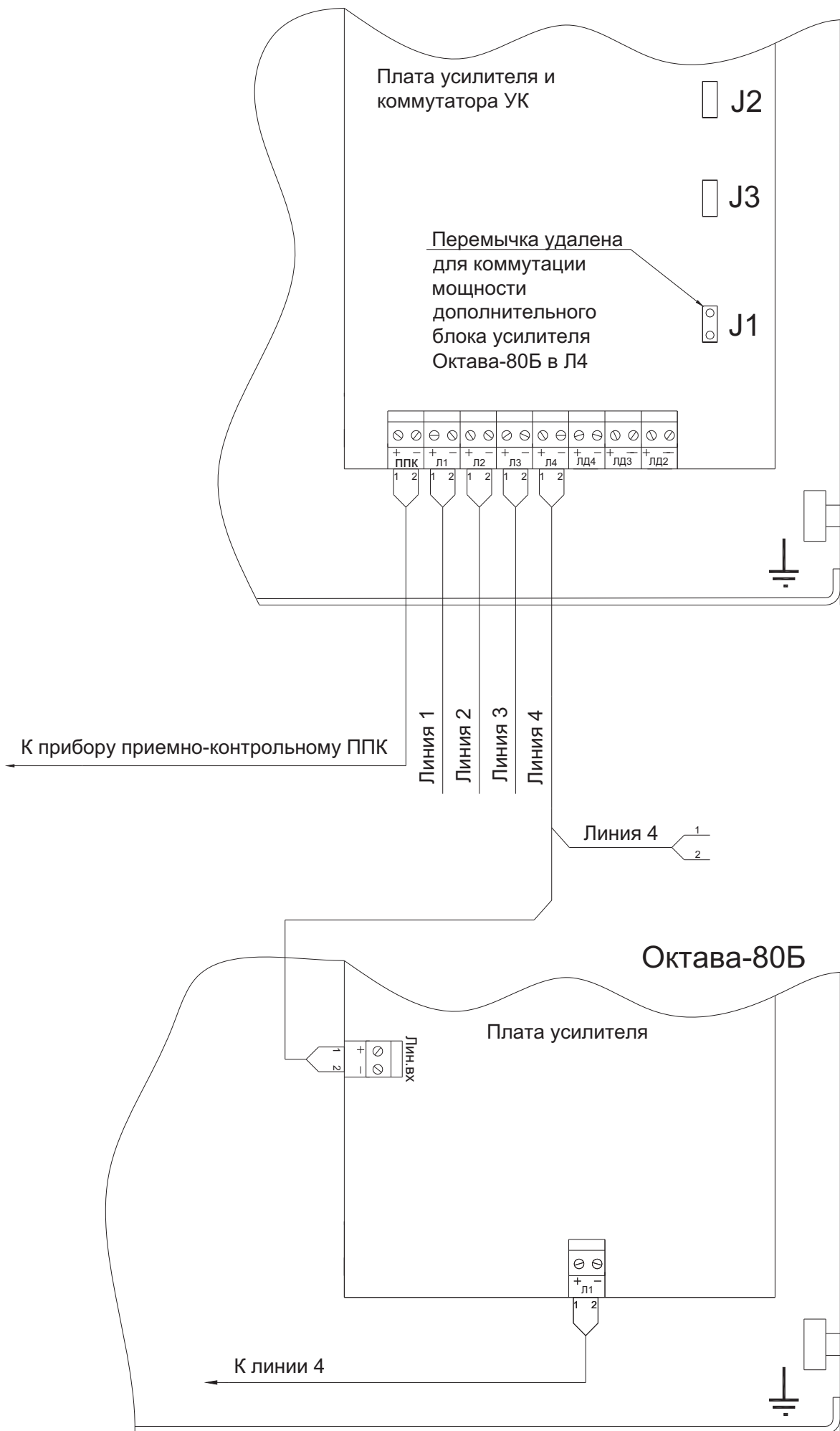
Схема подключения дополнительного усилителя мощности Октава-80Б, в качестве буферного.
