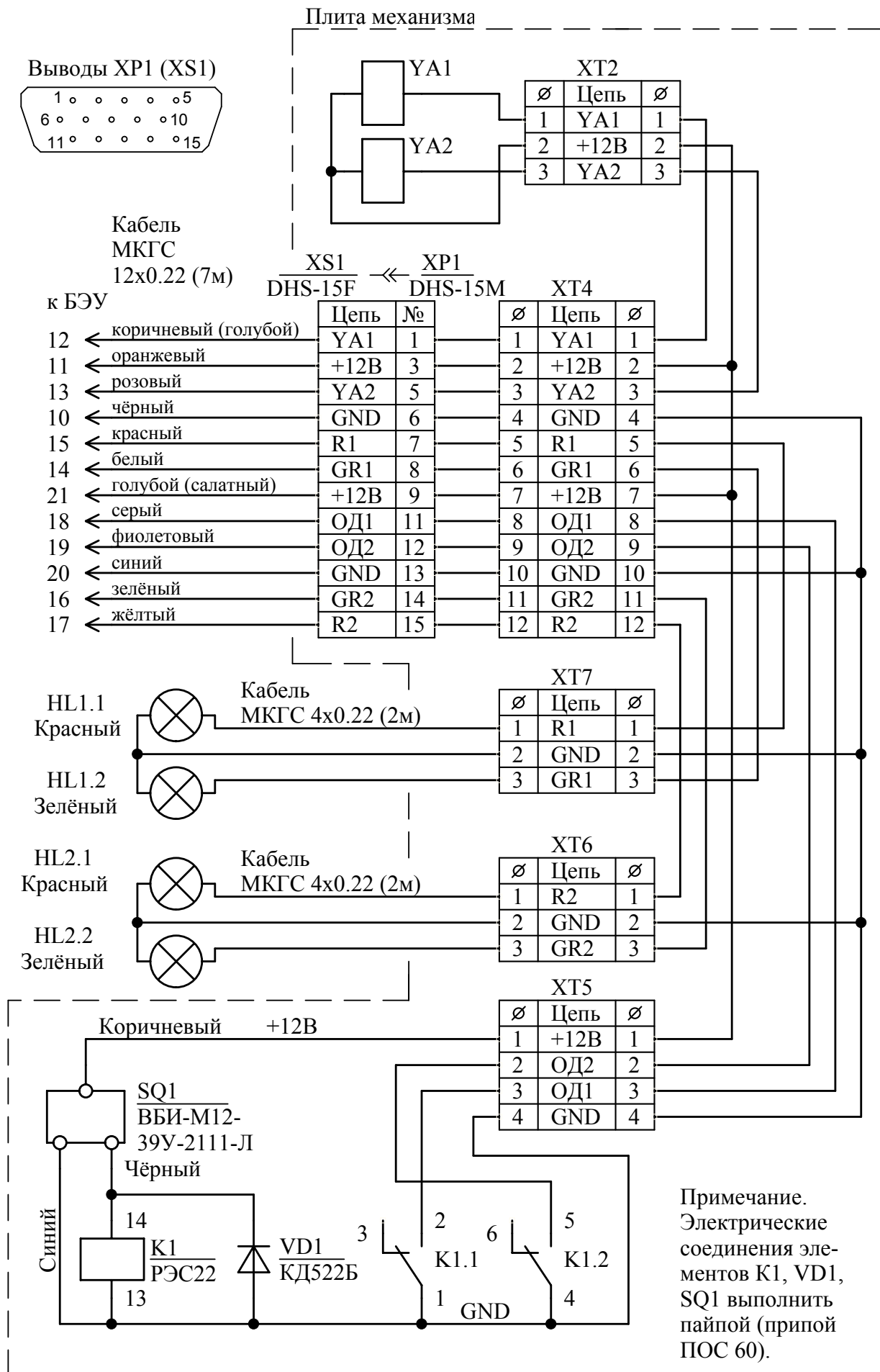
Схема электрическая принципиальная турникета ПР1 (Лист 2)
