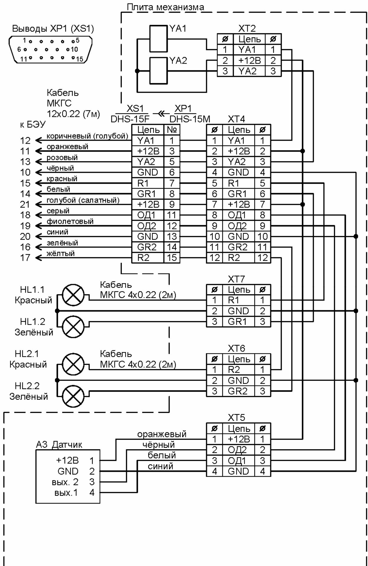
Схема электрическая принципиальная турникета ПР1 со счетчиком (Лист 2)
