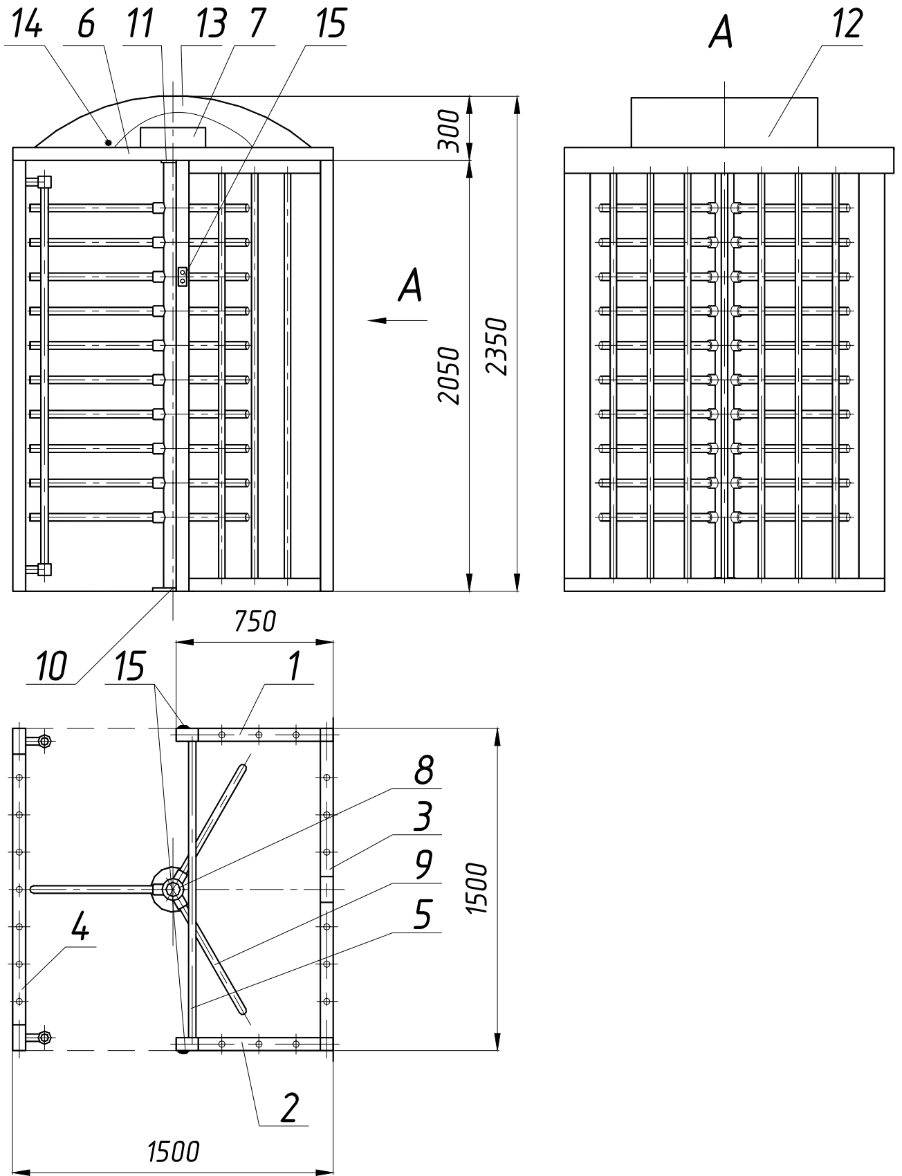
Габаритные размеры турникетов «Ростов-Дон ПР1»
