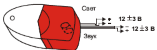
Рис.2 Схема подключения ПКИ-СП12.
