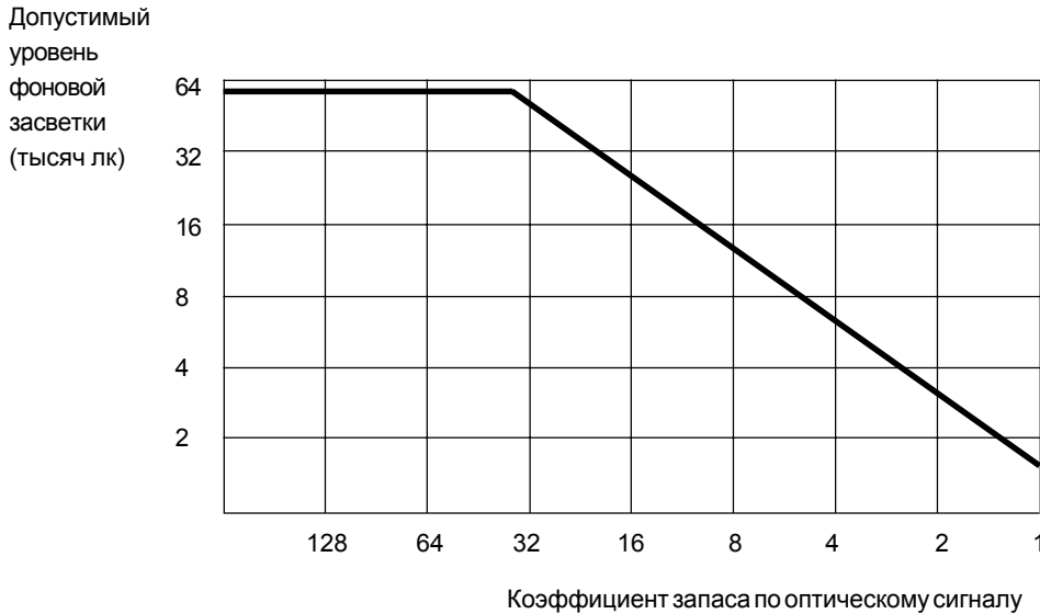
Зависимость допустимого уровня фоновой засветки от коэффициента запаса
