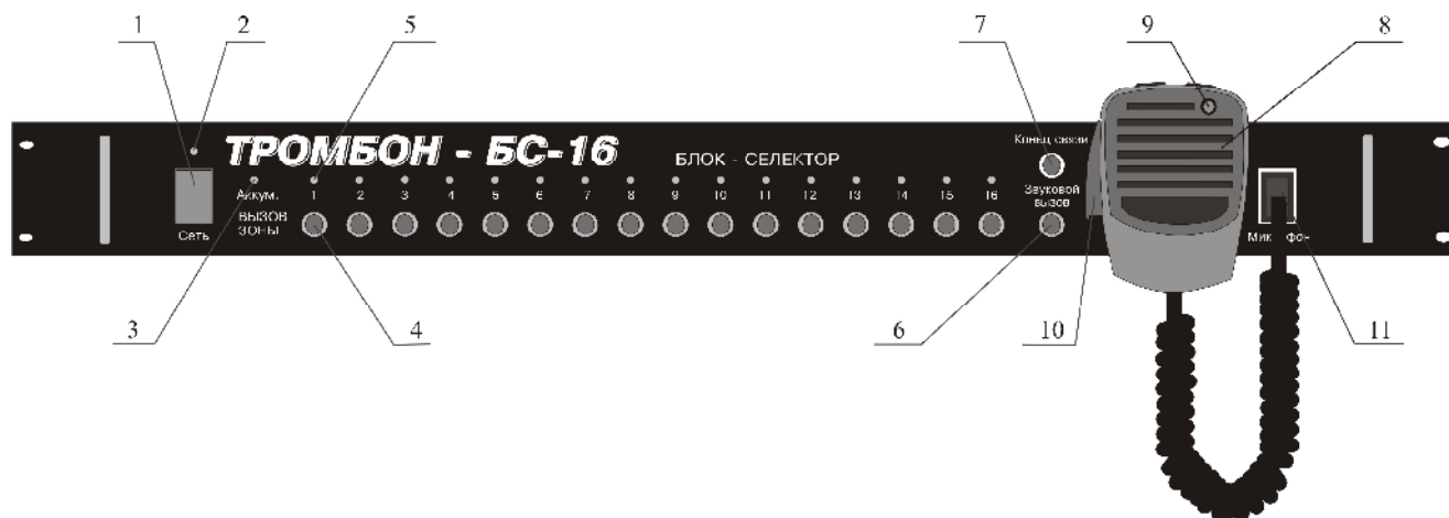
Рисунок 2 - Внешний вид Блока-селектора «Тромбон - БС-16» .
