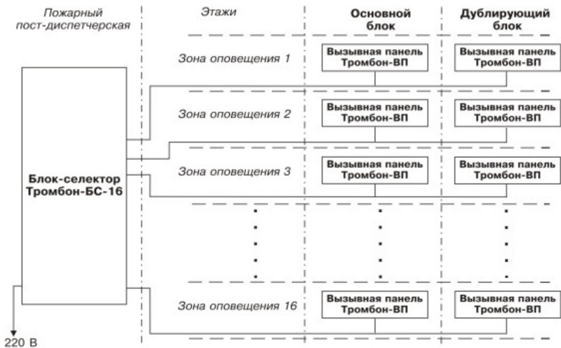
Рис. 1 Схема соединения между главным и периферийными блоками Устройства селекторного.
