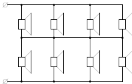
Схема подключения восьми акустических систем 4 Ом, 3Вт. Выходная мощность на динамиках 1,85 Вт.
