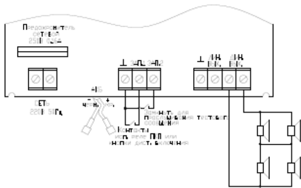
Варианты подключения акустических систем с акустическим сопротивлением 2 Ом.
