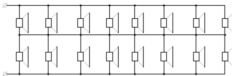
Схема подключения шестнадцати акустических систем 8 Ом, 3Вт. Выходная мощность на динамиках 1,5 Вт.
