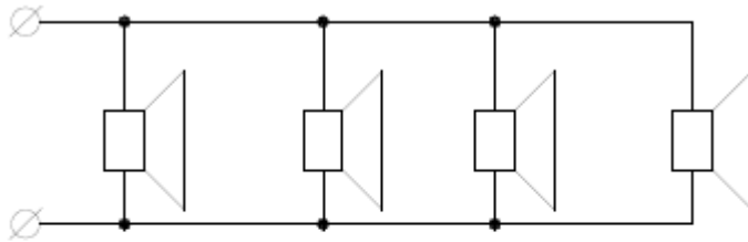
Схема подключения четырех акустических систем 8 Ом, 8-10Вт. Выходная мощность на динамиках 6 Вт.
