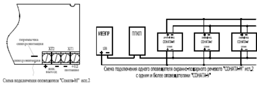
Схема подключения оповещателя «Соната-М» исп.2
