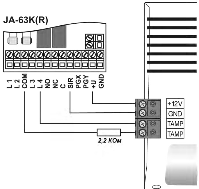
Рис. 2 пример подключения сирены к контрольной панели JA-63K(R)
