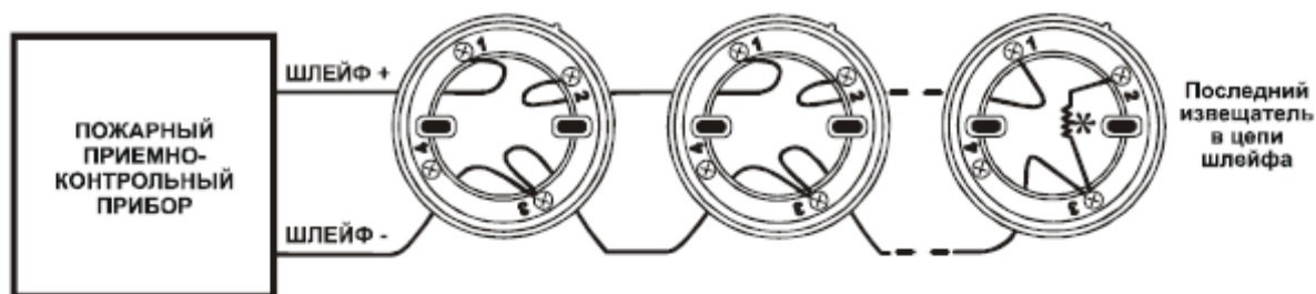
Схема подключения извещателей к приемно-контрольному прибору (без ВУОС)
