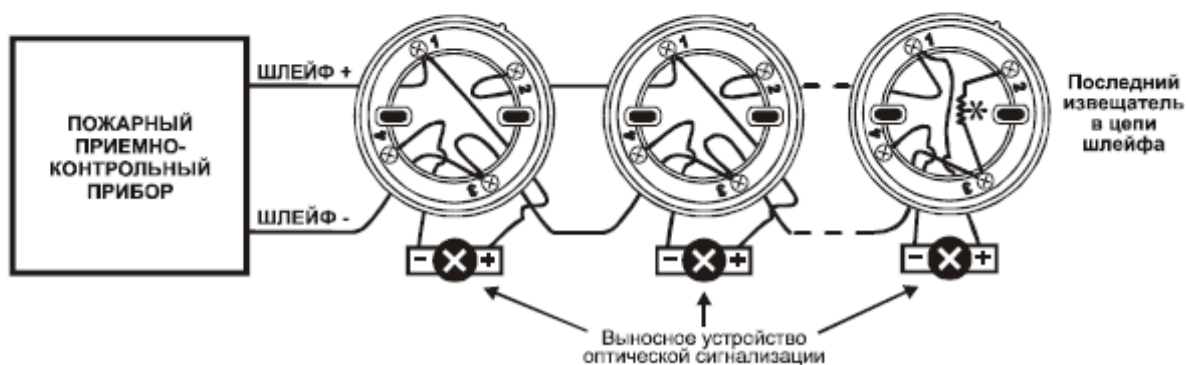
Схема подключения извещателей к приемно-контрольному прибору (с ВУОС)
