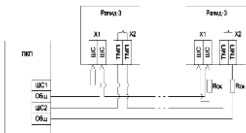
Рис.1 Схема подключения извещателя
