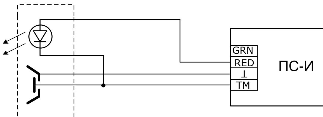
Считыватель ключей Touch Memory
