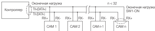
<Полудуплексная передача RS-485>
