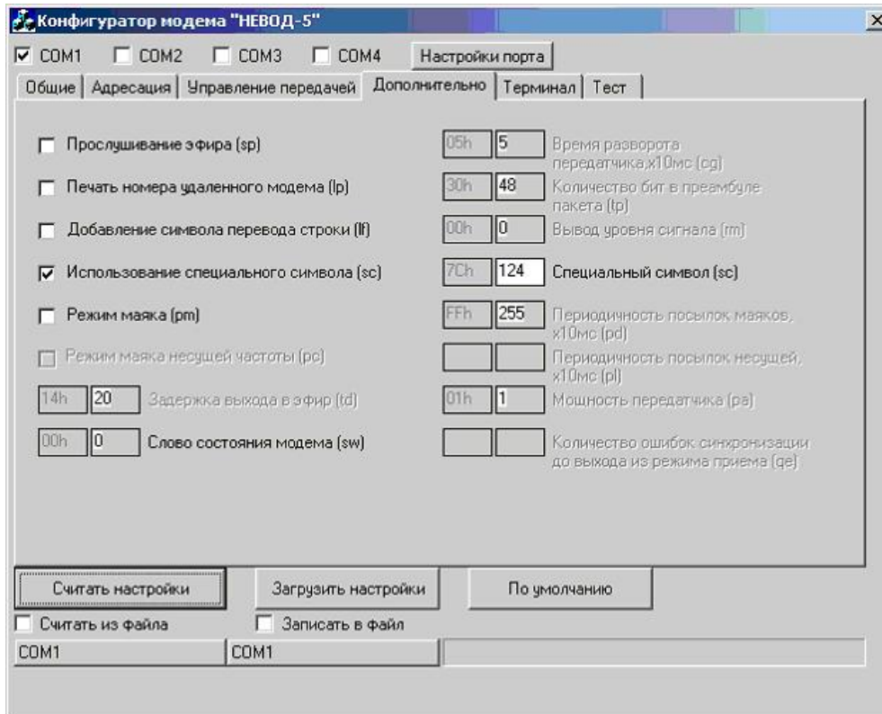
Рис.5 Вкладка «Дополнительно»
