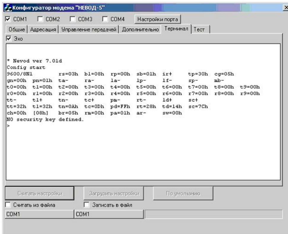
Рис.6 Вкладка «Терминал»
