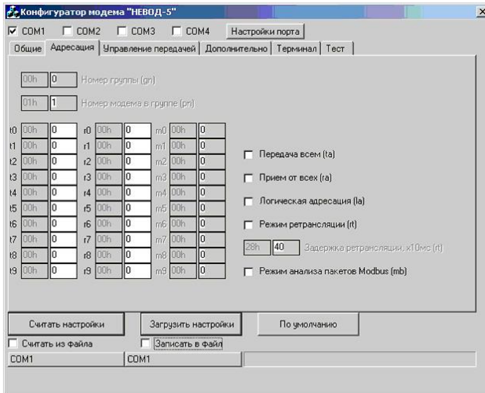
Рис.3 Вкладка «Адресация»
