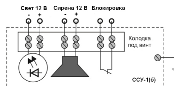
Рис.1 Схема подключения оповещателя ССУ-1(б)
