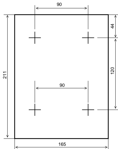
Рисунок 2. Габаритно-установочные размеры
