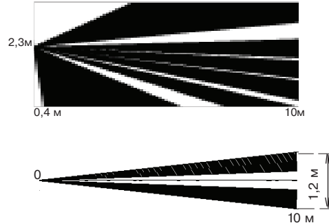
Рисунок 1 - Диаграмма зоны обнаружения
