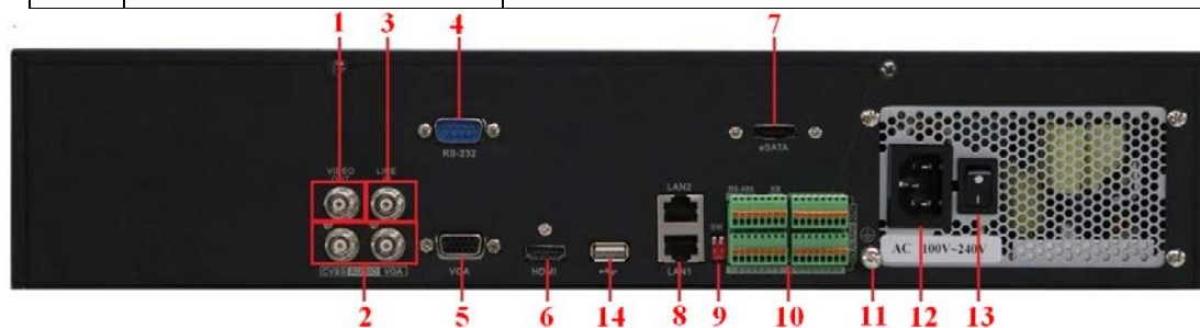
Цифровой видеорегистратор BestNVR-3204 IP
