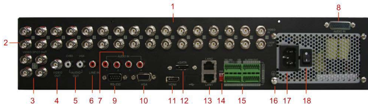
Рисунок 2 Цифровой видеорегистратор BestDVR-1604Hybrid-S
