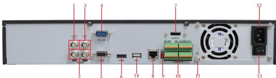
Рисунок 3 Цифровой видеорегистратор BestNVR-804/1604 IP
