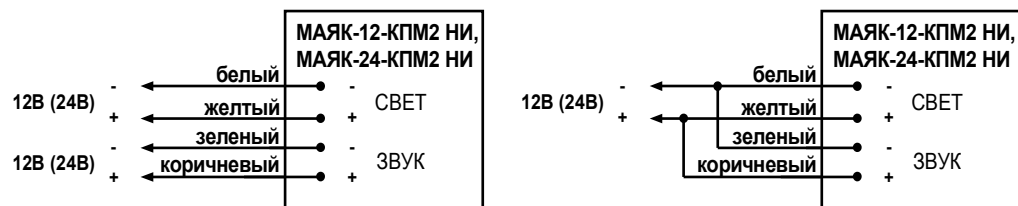
Рис.1. Схема подключения.
