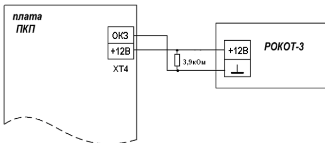
Рис.4 Схема подключения к прибору «Кварц» вариант 2
