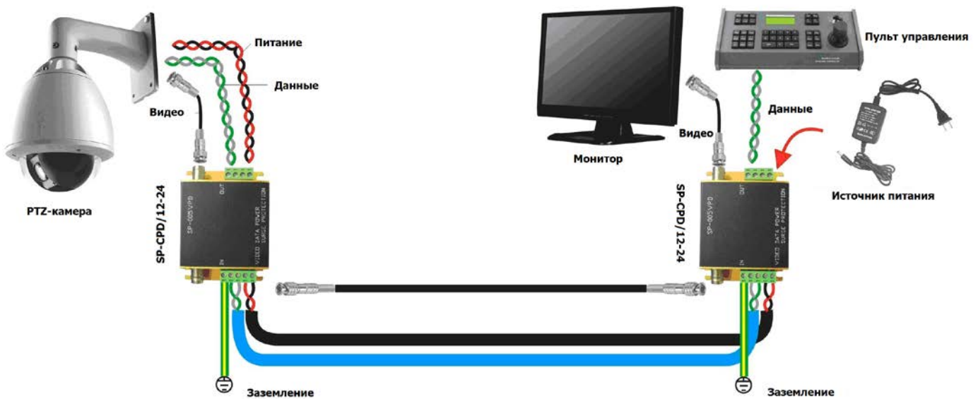
Рис. 3 Подключение SP-CPD/12-24
