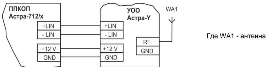
Рисунок 7. Схема подключения ППКОП «Астра-712/Х»
