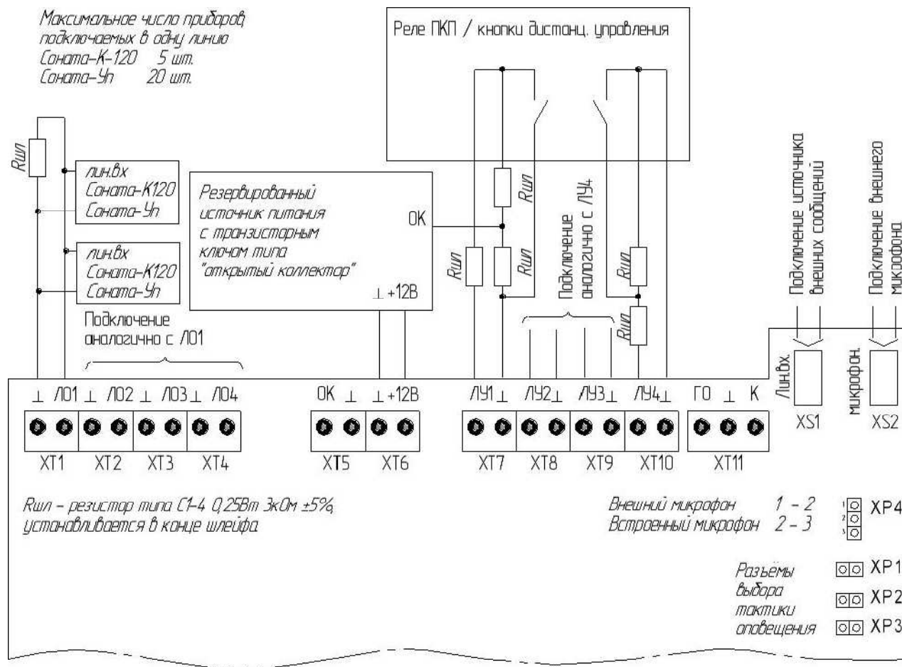
Рисунок-1 Схема внешних подключений прибора Сوناتа-ПУ с вариантом реализации запрета трансляции с линейного входа (см. п.п. 4.2) при питании прибора Сوناتа-ПУ от резервированного источника питания с транзисторным ключом типа «открытый коллектор»
