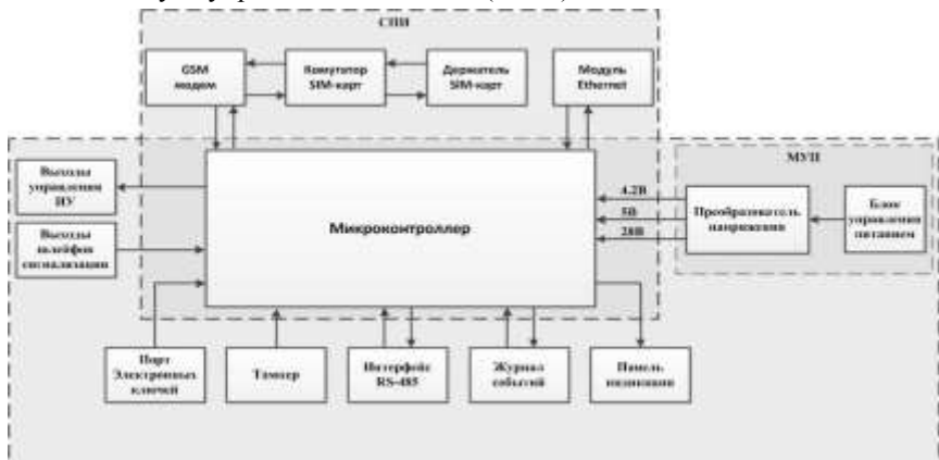
Рис. 1. Функциональная схема контроллера
