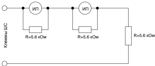
Схема включения пожарных извещателей со стратегией Тепловой
