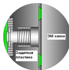
Замок в положении - закрытый
