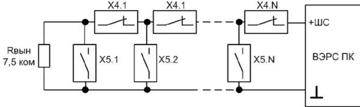
Рисунок Б5. Схема включения линейных дымовых извещателей ИПДЛ-Д-II/4Р.
