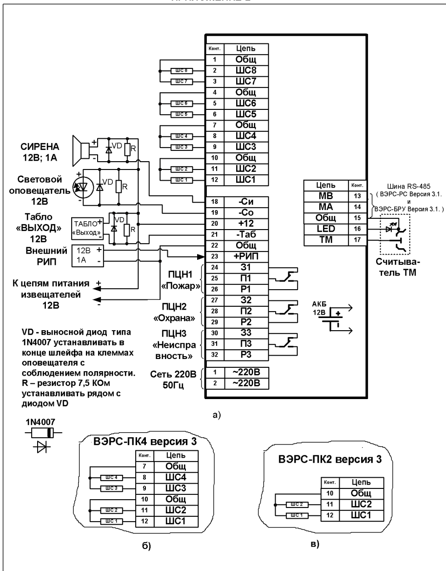
Рисунок. Б1. Схемы внешних соединений приборов ВЭРС-ПК(8,4,2) ТРИО-М.
