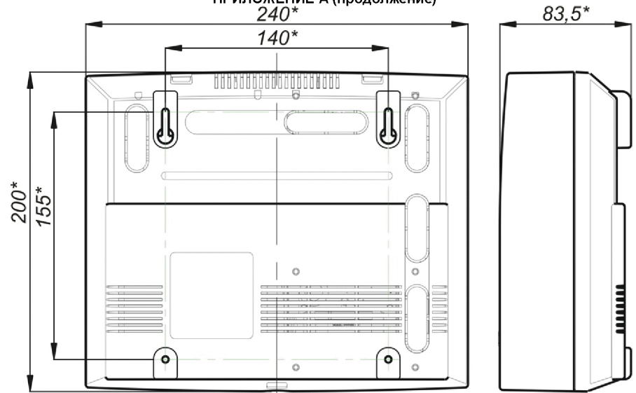
Рисунок А2. Габаритные и установочные размеры приборов ВЭРС-ПК(8,4,2) ТРИО-М.
