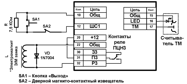
Рисунок Б8. Схема организации Точки доступа.
