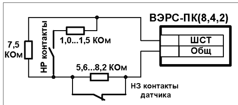
Рисунок Б7. Схема включения технологических датчиков в ШСТ. НР - нормально разомкнутые контакты датчика НЗ - нормально замкнутые контакты датчика
