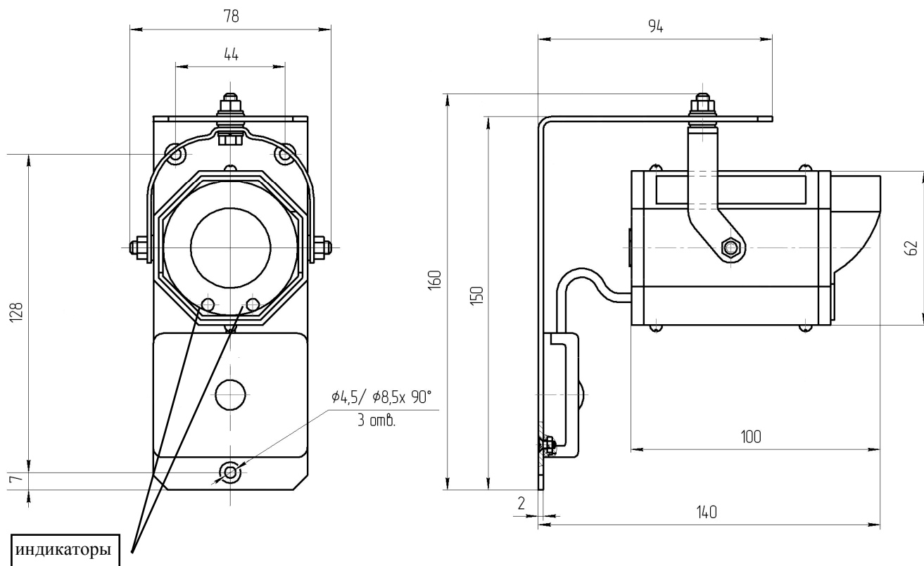
Рис.1а Блок излучателя БИ
