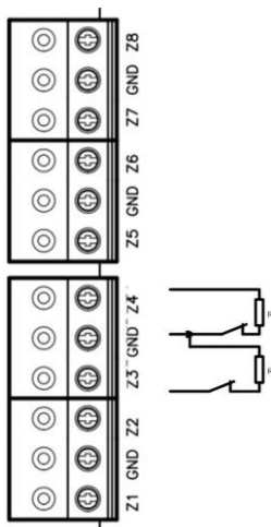
Рис.10. Подключение дверного контакта
