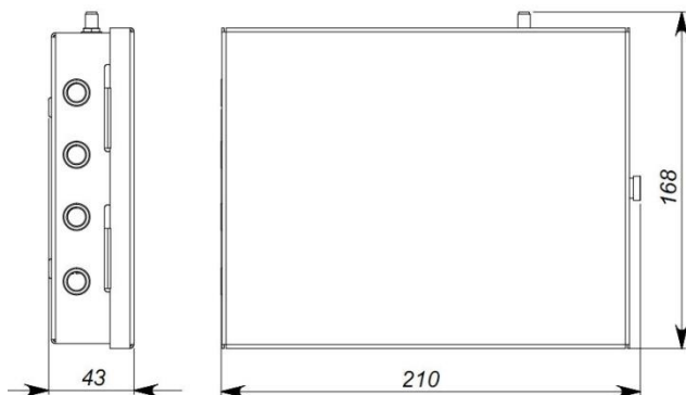
Рис 6. Габаритные размеры
