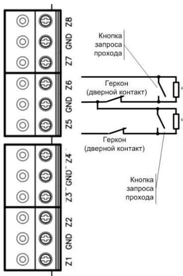
Рис.11. Подключение комбинированного шлейфа
