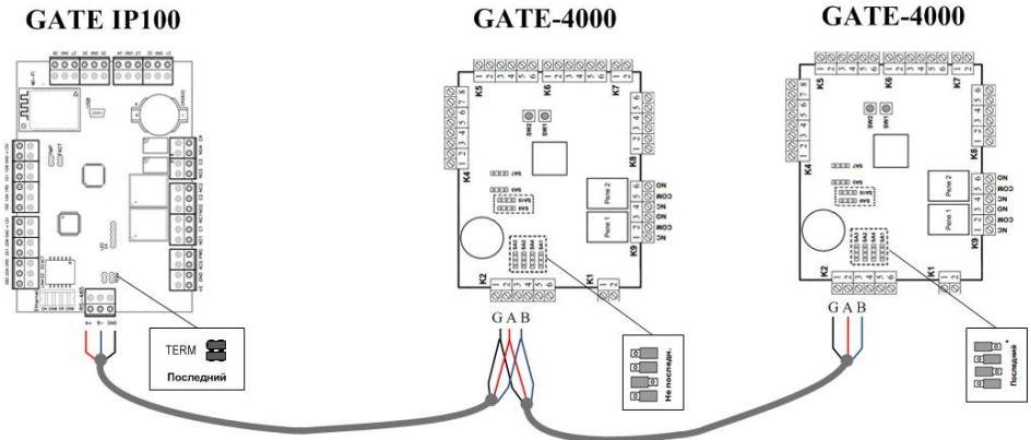
Рис.17. Контроллер Gate-IP100 последний (первый) на шине данных
