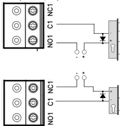
Рис.13. Подключение замков
