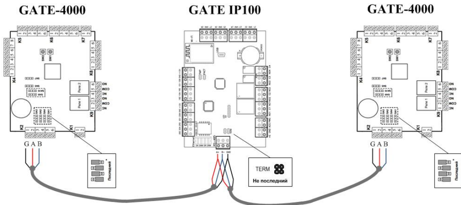
Рис.16. Контроллер Gate-IP100 центральный на шине данных
