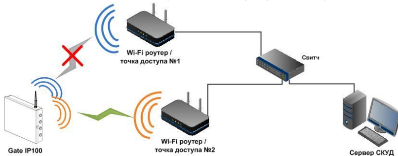
Рис 5. Работа с несколькими Wi-Fi точками доступа
