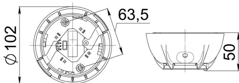
Рисунок 2 – Монтажная схема.
