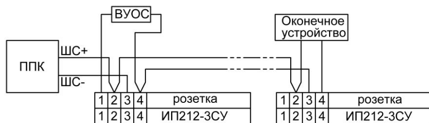
Рисунок 1 – Схема включения.
