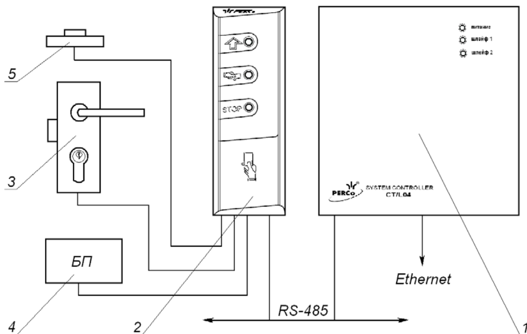
Рисунок 1. Функциональная схема
