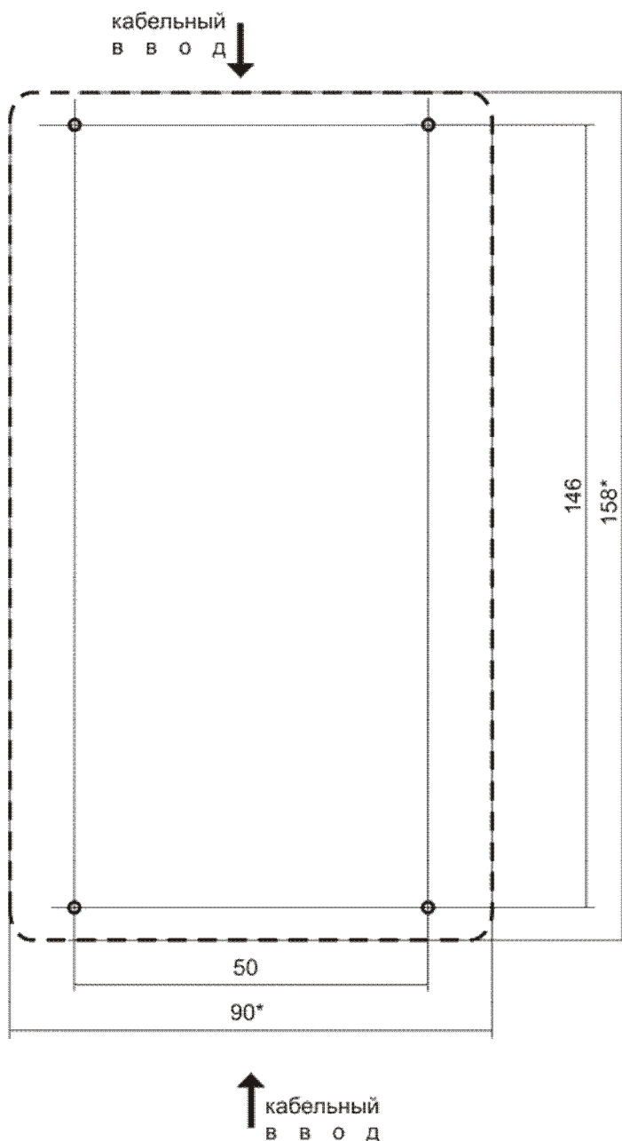
Приложение 1. - Разметка крепления барьера Толмач «АБИЗ»
