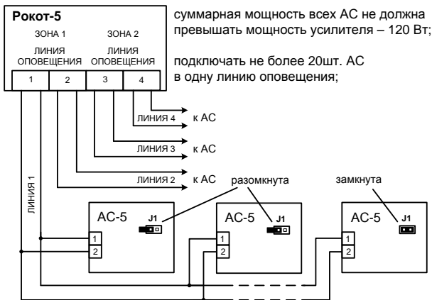
Рис.2 Схема подключения АС-5 к Рокот-5 ПУО и Рокот-5 УМ
