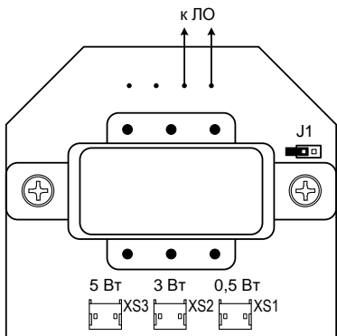
Рис.1 Плата АС-5
