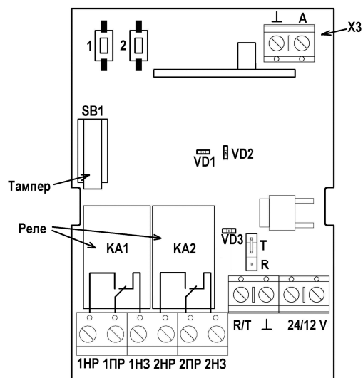
Рисунок 1 – Плата приёмника Лидер-4
