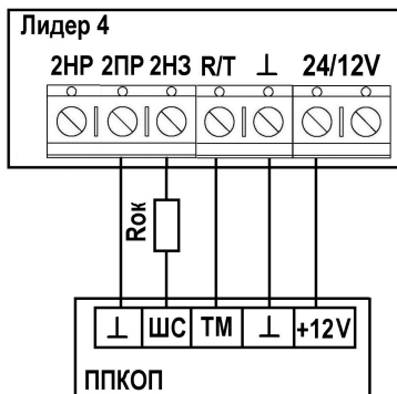
Рисунок 3 – Схема подключения блока приёмника Лидер-4 к приемно-контрольному прибору (ППКОП)
