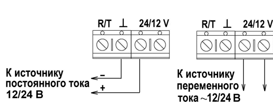
Рисунок 2 – Схемы подключения приёмника Лидер-4 к источнику электропитания
