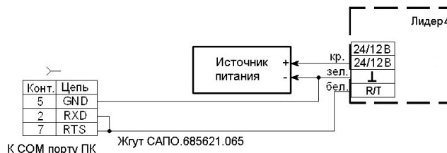
Рисунок 5 – Схема подключения блока приёмника Лидер-4 к СОМ порту персонального компьютера (ПК). Жгут подключения поставляется отдельно.
