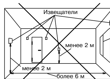
Рисунок 9 – Нерекомендуемые места установки извещателя
