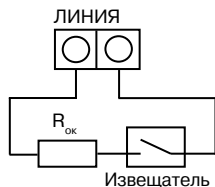
Рисунок 2 – Схема подключения датчика перемещения охраняемой конструкции
