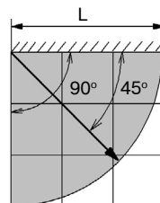
Рисунок 3 – Диаграмма зоны обнаружения АК канала
