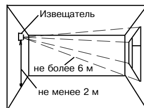
Рисунок 6 – Установка извещателя на противоположной стене
