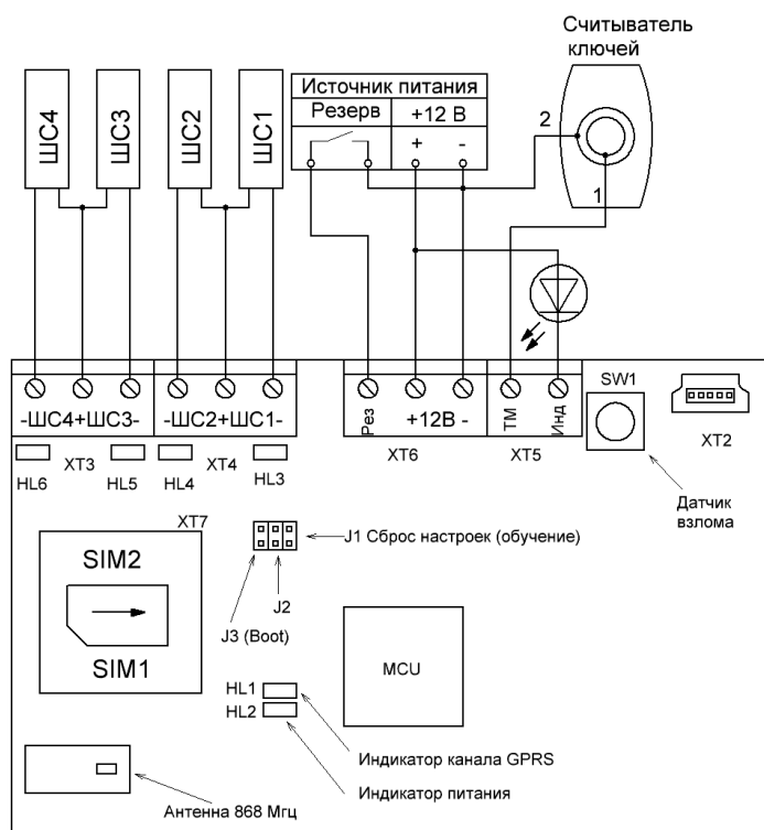
Рисунок 2.3. Назначение разъемов прибора
