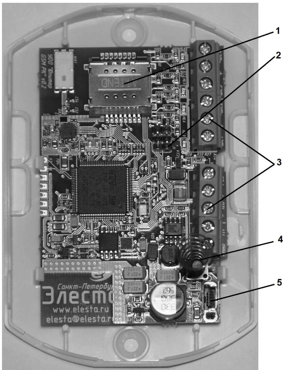
Рисунок 2.2. Вид прибора с открытой крышкой
