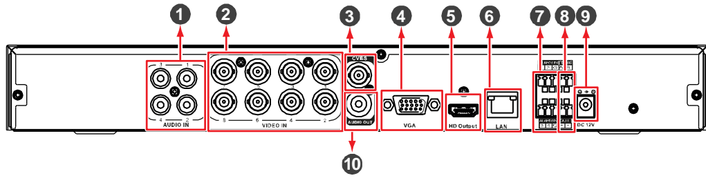
Рис. 1-2 Описание и разъемы задней панели 4-канального и 8-канального DVR
